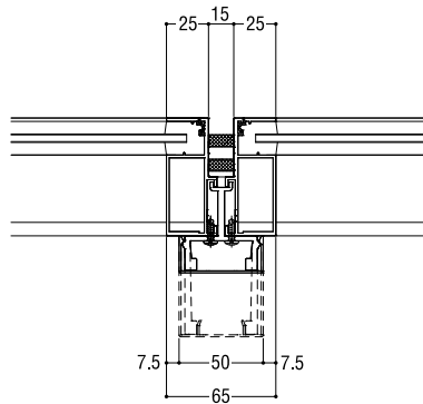
FIX窓 (20mm) - FIX窓 (20mm)
